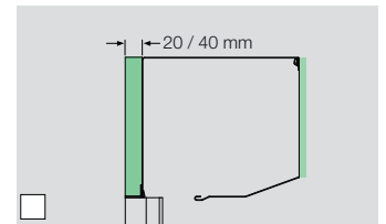
Kastendämmung rückseitig für Abstand-Führungsschiene mit 20 oder 40 mm
